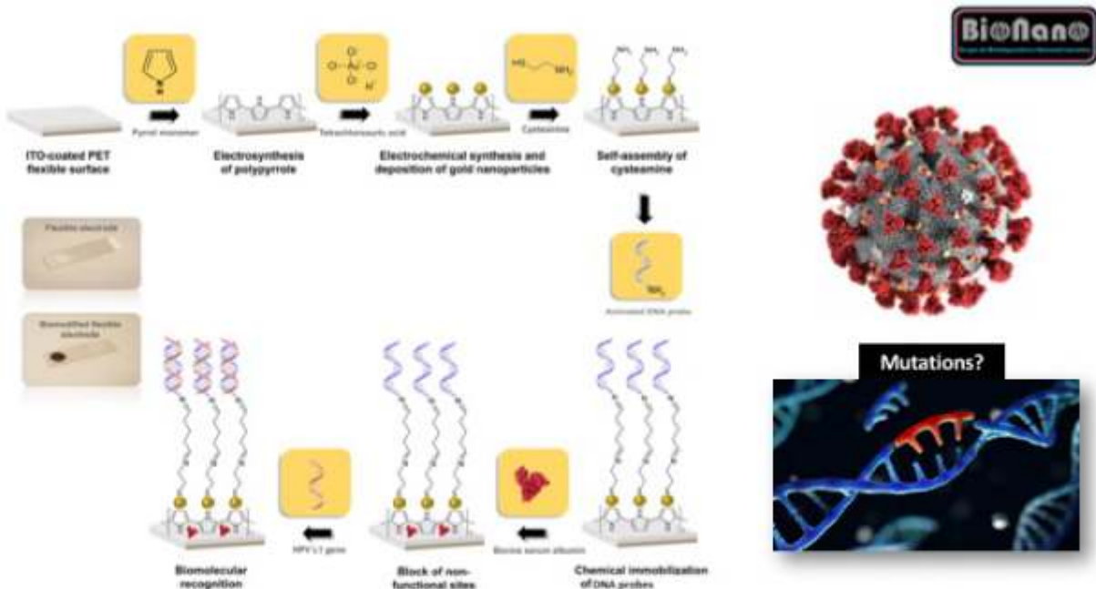
Representação esquemática das etapas de montagem do biossensor flexível baseado em polipirrol (PPy), nanopartículas de ouro (AuNPs), cisteamina (Cys), sondas de DNA aminadas e albumina sérica bovina (BSA).
